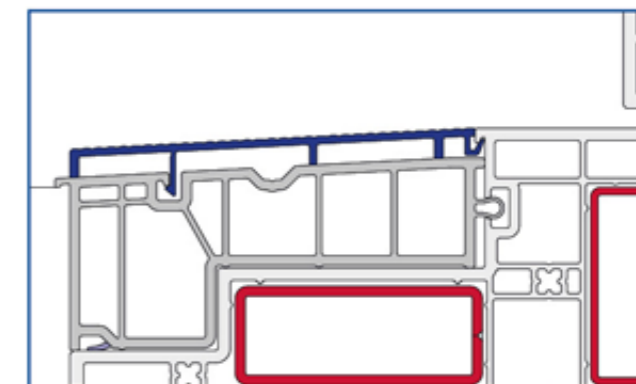
Standard küszöb
