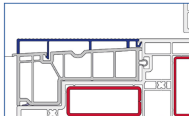
Akadálymentes küszöb
