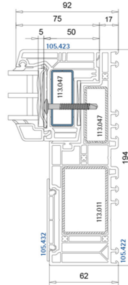
Fix szárny kiüvegezve szerelve
